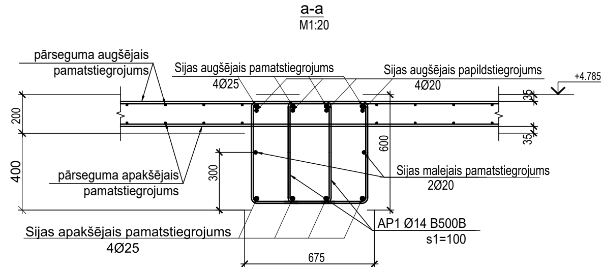
Dz/betona sija S-2
