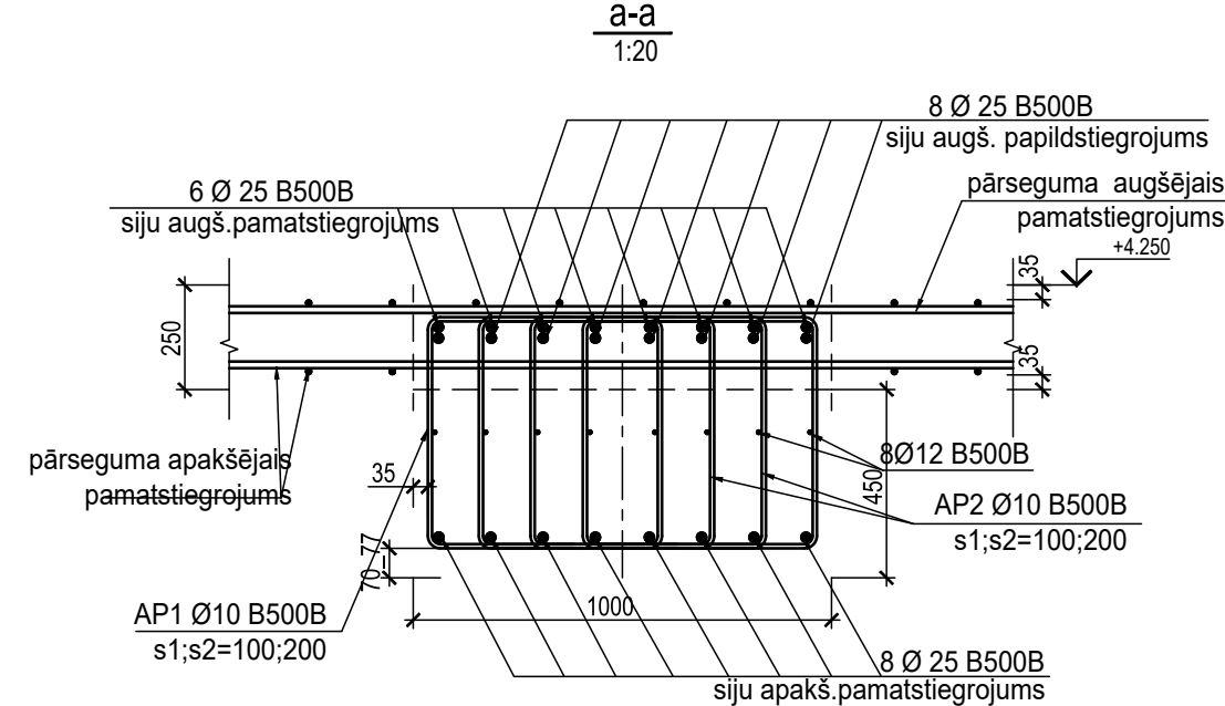
Dz/betona sija S-9
