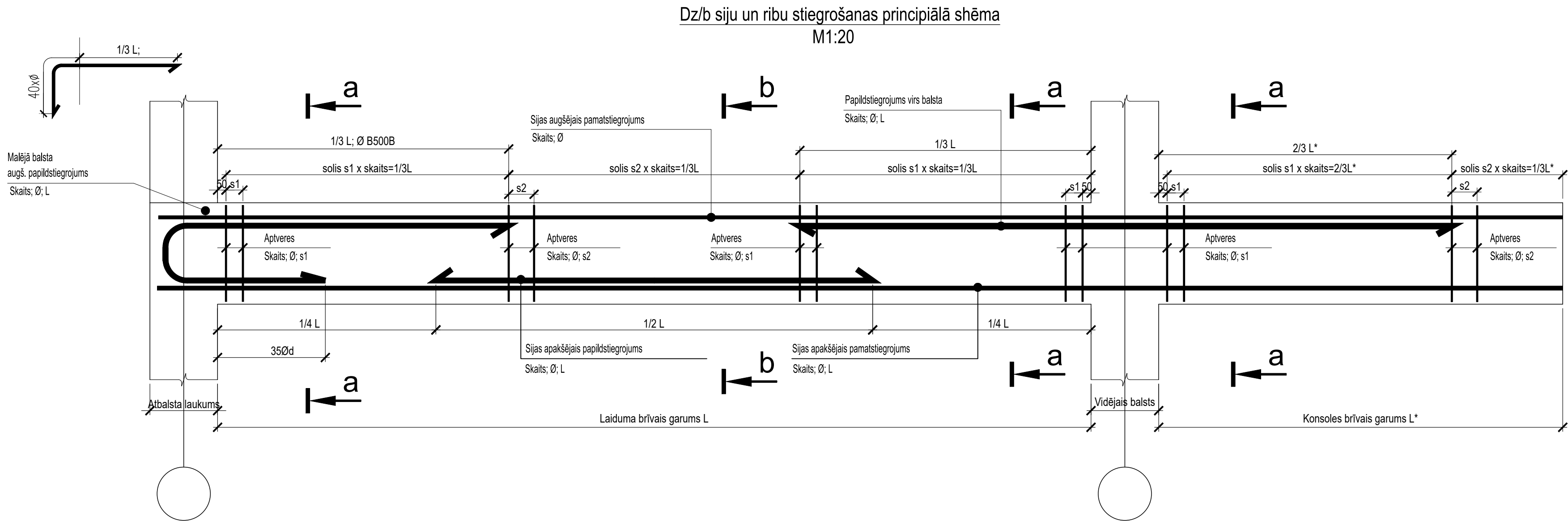
Dz/betona sija S-9
