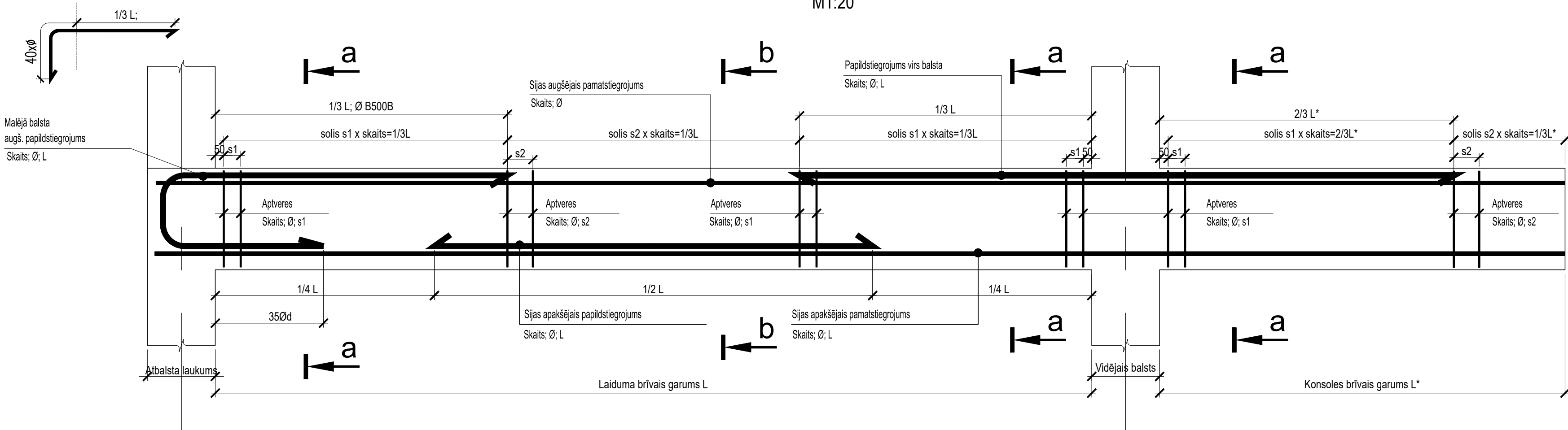
Dz/betona sija S-10 a-a, b-b 1:20
