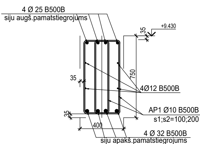
Dz/betona sija S-10 a-a, b-b 1:20
