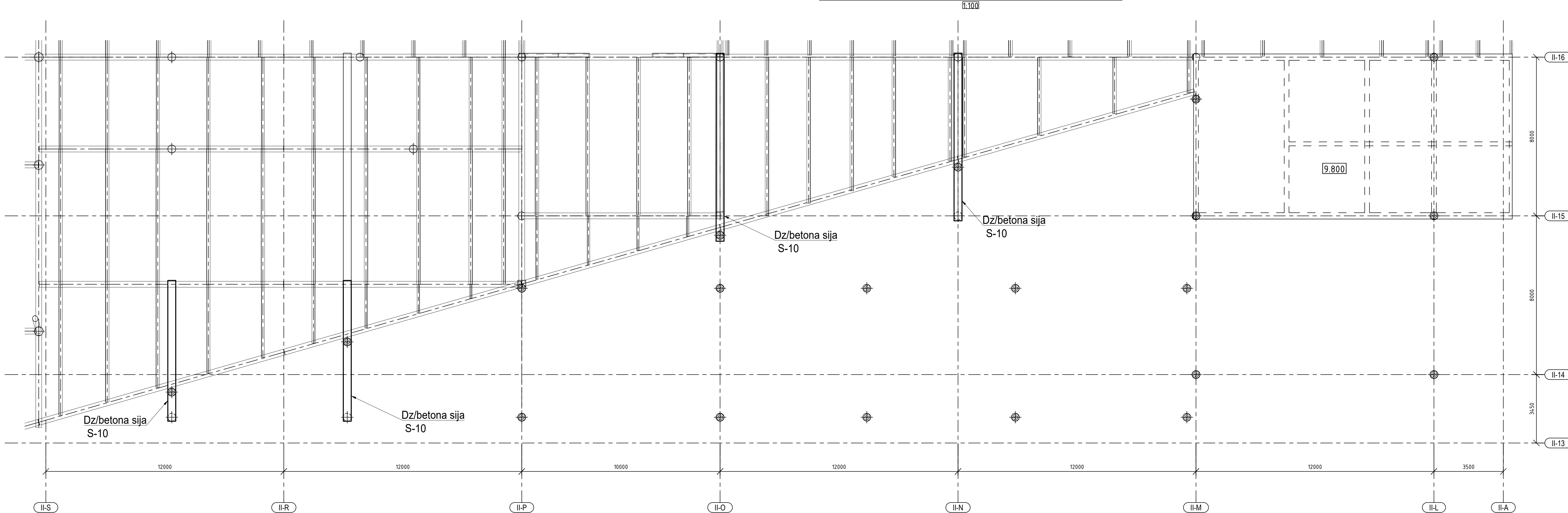
Dz/b siju un ribu stiegrošanas principiālā shēma M1:20
