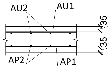
Stiegrojuma principiālais izvietoējums plātnē
