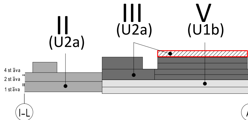
Dalījuma shēmas griezumam
