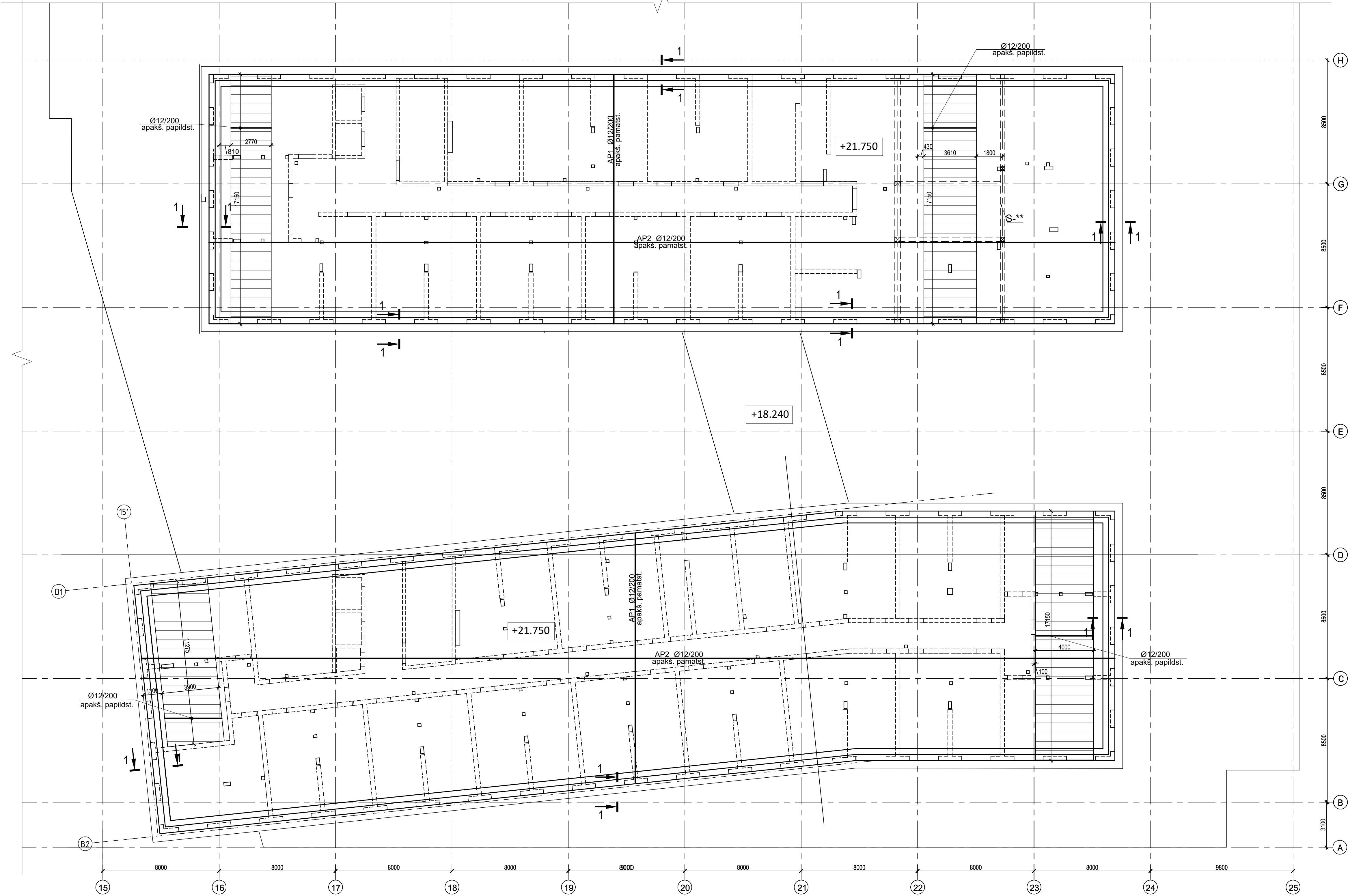
Pārseguma uz atz. +21.750 apakšējais stiegrojums 1:150
