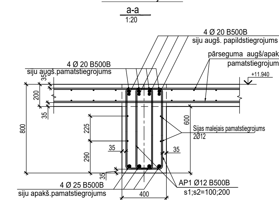
Dz/betona sija S-5
