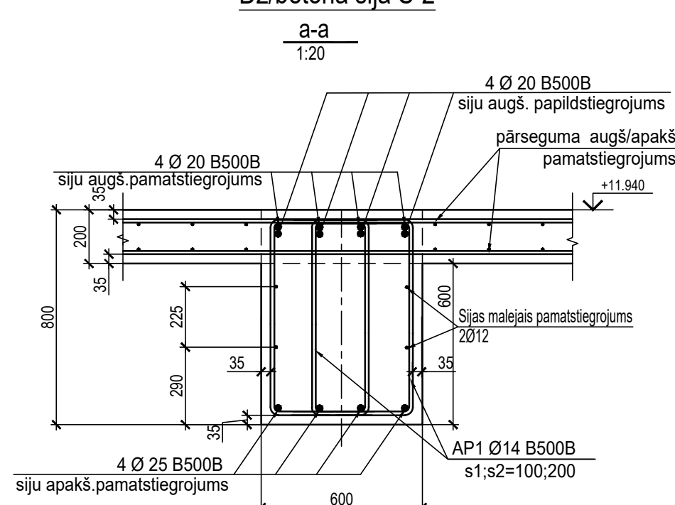
Dz/betona sija S-2
