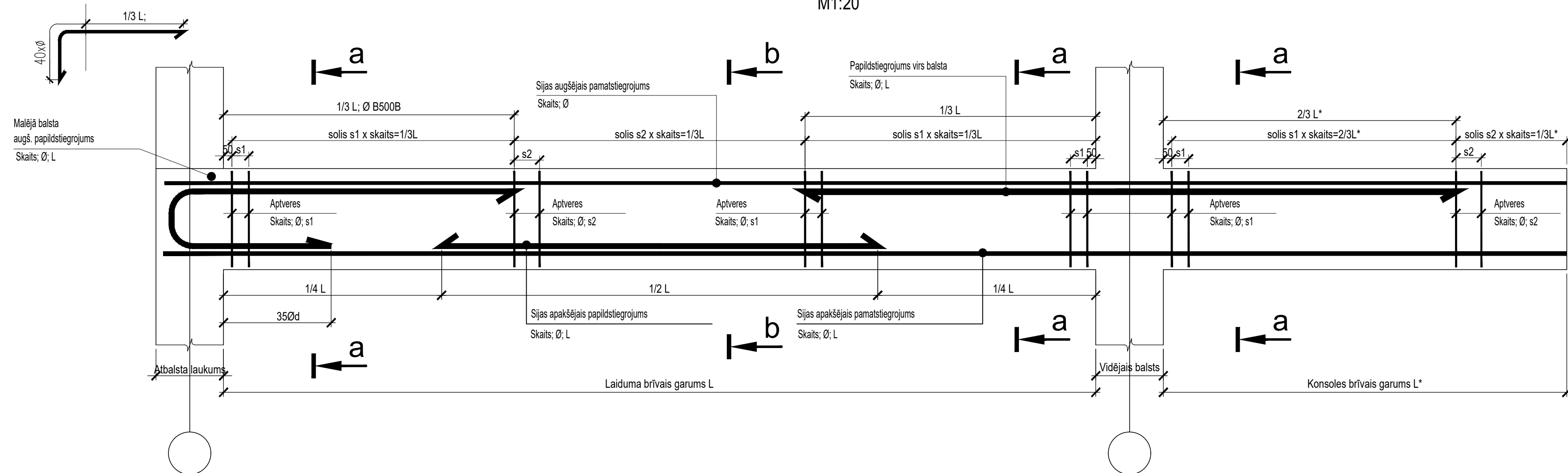
Dz/betona sija S-1
