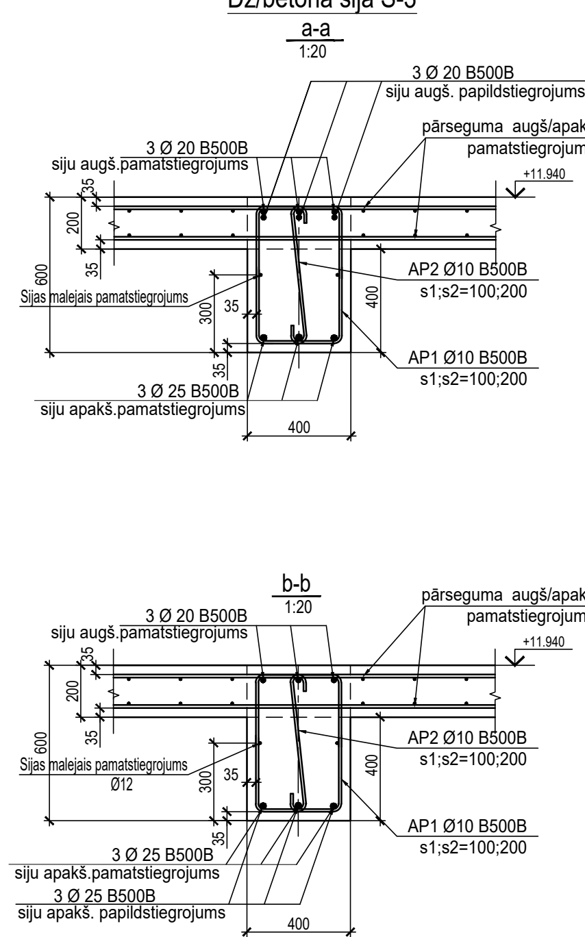
Dz/betona sija S-3
