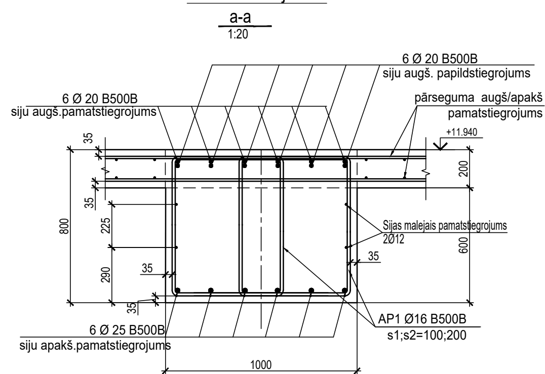
Dz/betona sija S-1
