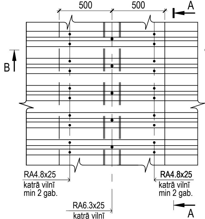
"Lokšņu stiprinājuma principiālais mezglis"
