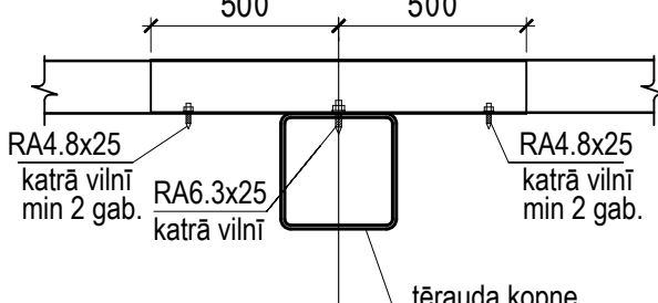
B-B
