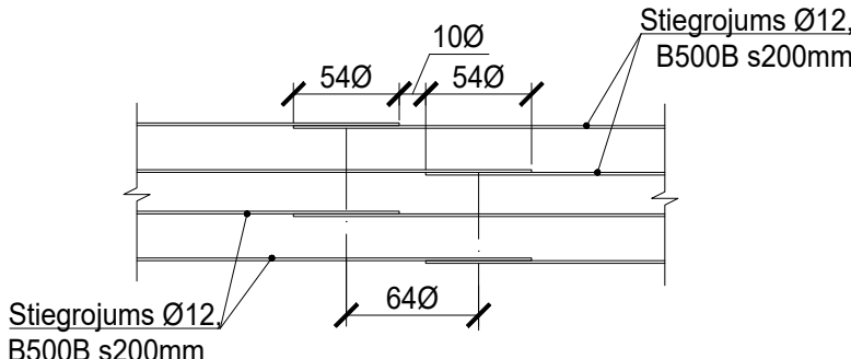
Pamatstieģrojuma pārlaiduma mezgls
