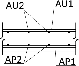
Stiegrojuma principiālais izvietojums plātnē
