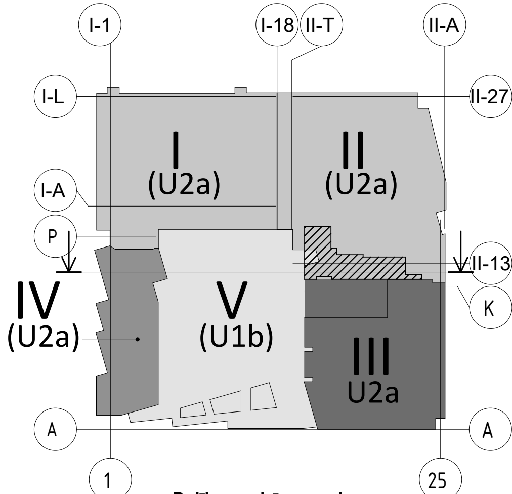
Dalījuma shēmas griezumā
