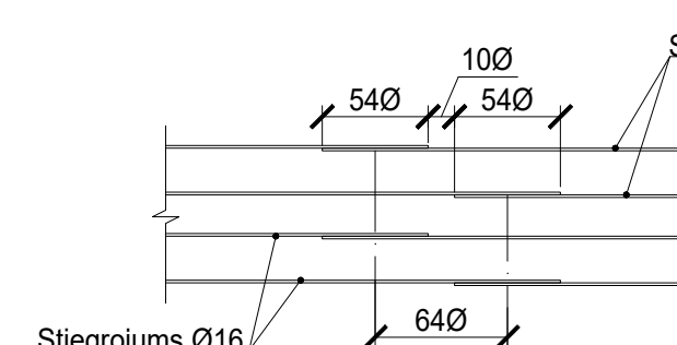
Pamatstieģrojuma pārlaiduma mezgls
