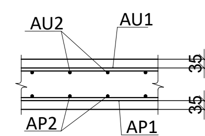
Stiegrojuma principiālais izvietojums plātnē
