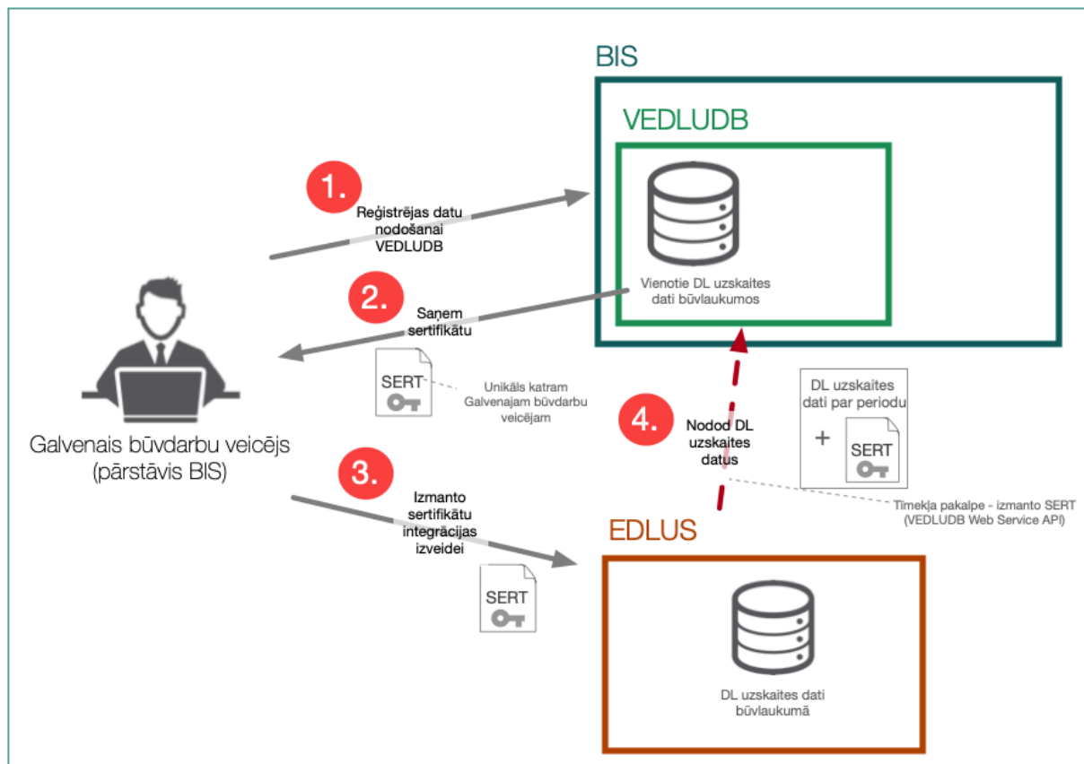
Attēls nr. 1 Būvlaukuma reģistrācija datu nodošanai no EDLUS uz VEDLUDB
