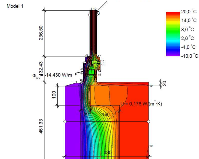
Loga un ārējas mezgls
