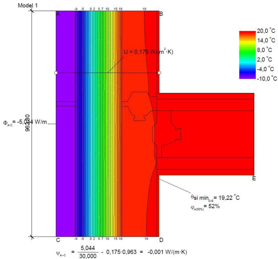
Pārseguma un ārējas mezgls
