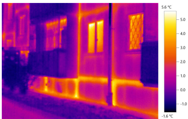
15.attēls. Ēkas ziemeļu fasāde
