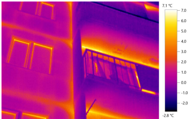
7.attēls. Termiskais tilts ārsiena/balkons
