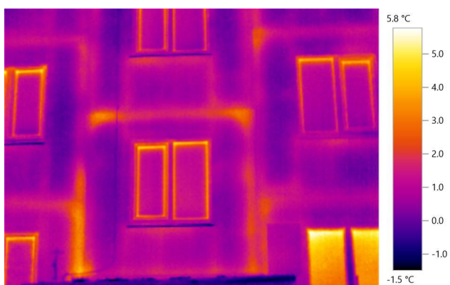
18.attēls. Paaugstināta virsmas temperatūra paneļu savienojuma vietās
