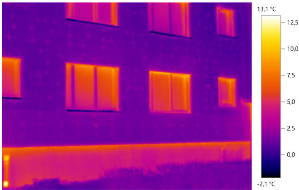
1. att. Ēkas fasāde (siltināta) un cokols (nesiltināts)
