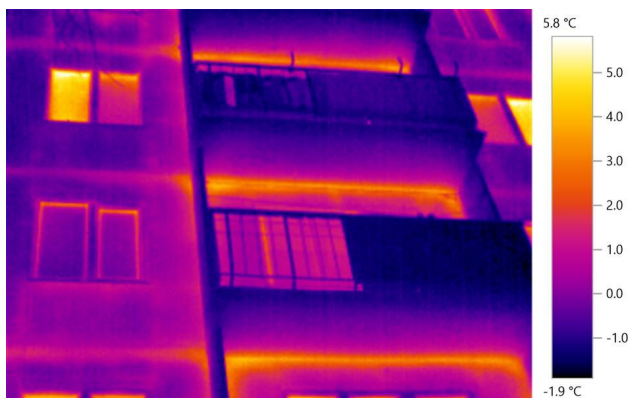
10.attēls. Termiskais tilts ārsiena/balkons
