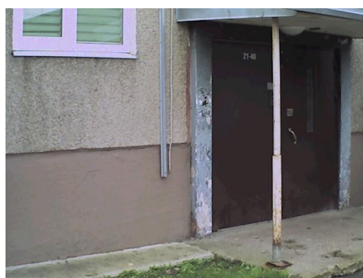
17.attēls. leejas bloks, termiskais tilts paneļu savienojuma vietā
