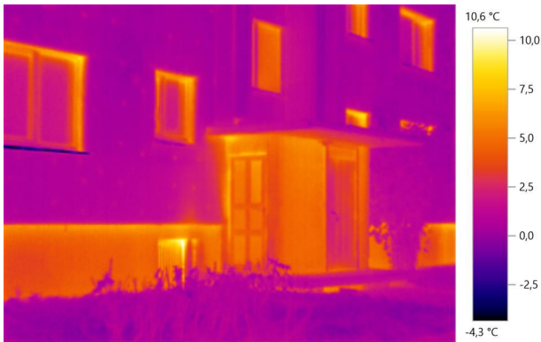
4.att. Ēkas ārsiena (termiskie tilti dībeļu vietās siltumizolācijā)
