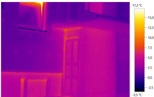
2.att. Ēkas ieejas mezgls un ārsiena (termiskais tilts)
