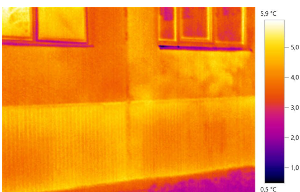
6. att. Ēkas cokols un ārsiena
