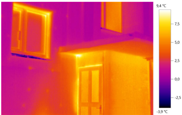
5. att. Ēkas ārsiena un ieejas mezgls
